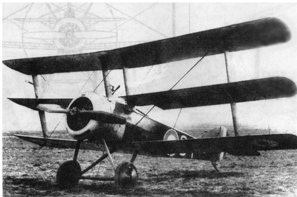
Сопвич Триплан (Sopwith Triplane), истребитель 1916 г. (компания «Сопвич Авиэйшн», Великобритания)
