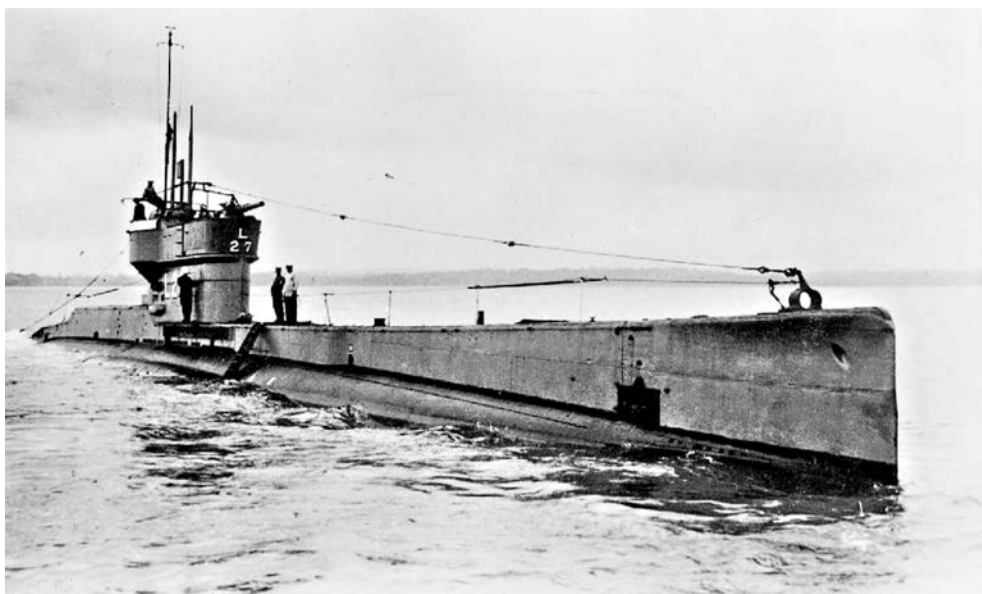
Британская подводная лодка класса L (HMS L. 27) 1919 г. (компания «Виккерс Лтд.»)
