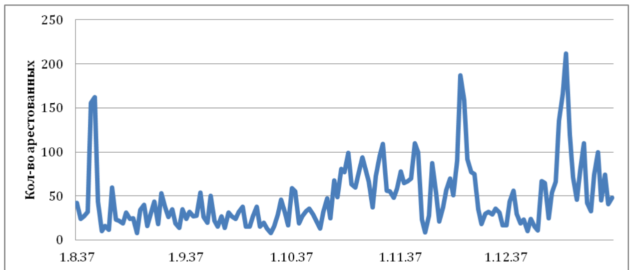
Рис. 14. Динамика арестов репрессированных в августе-декабре 1937 г. в Горьковской области.
