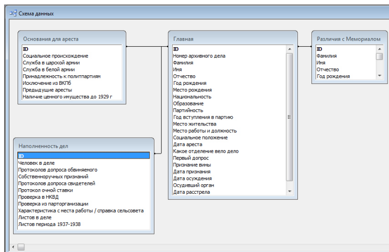
Рис. 5. Схема базы данных «Бутовский полигон» в Access.
