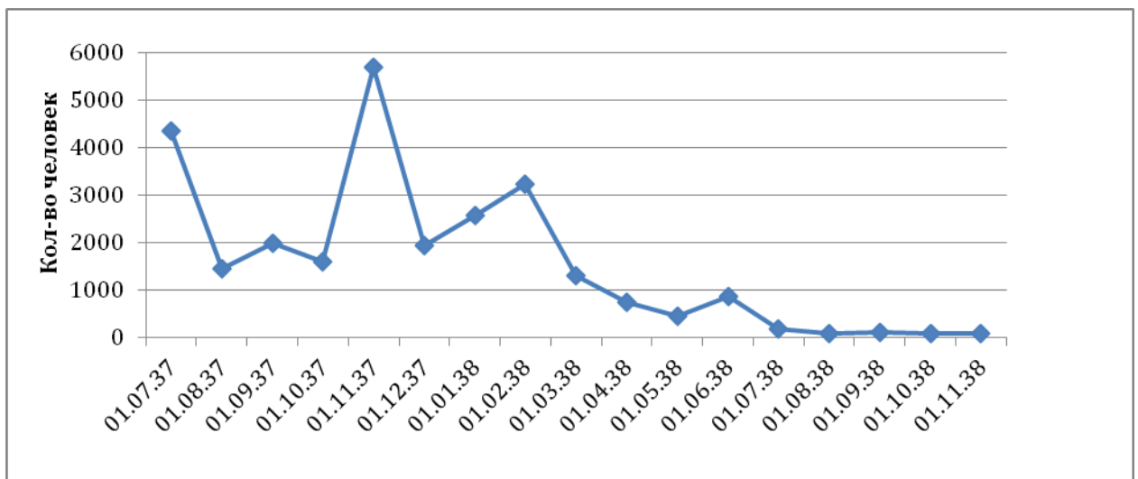
Рис. 6. Динамика арестов в Алтайском крае с июля 1937 г. по ноябрь 1938 г.
