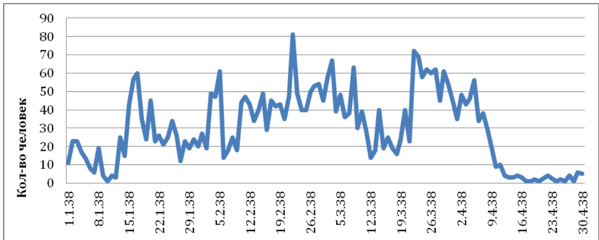
Рис. 20. Динамика арестов репрессированных в январе-апреле 1938 г. по дням.
