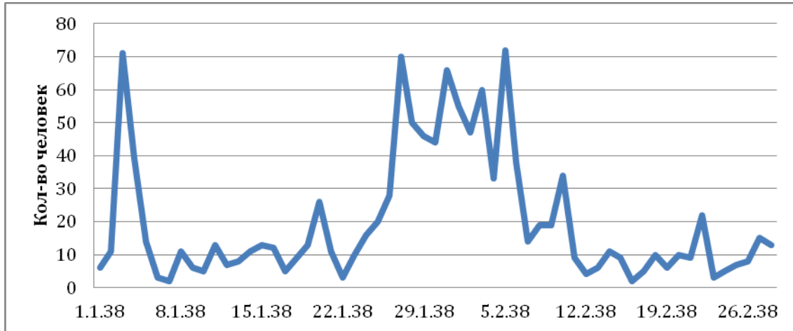
Рис. 16. Динамика арестов репрессированных в Горьковской области в январе-феврале 1938 г. по дням.
