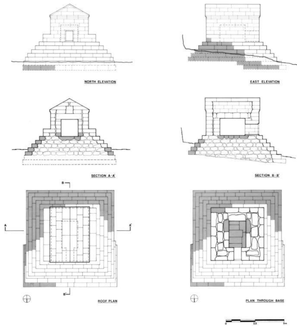
3.23 Сарды, «гробница-пирамида», варианты реконструкций
