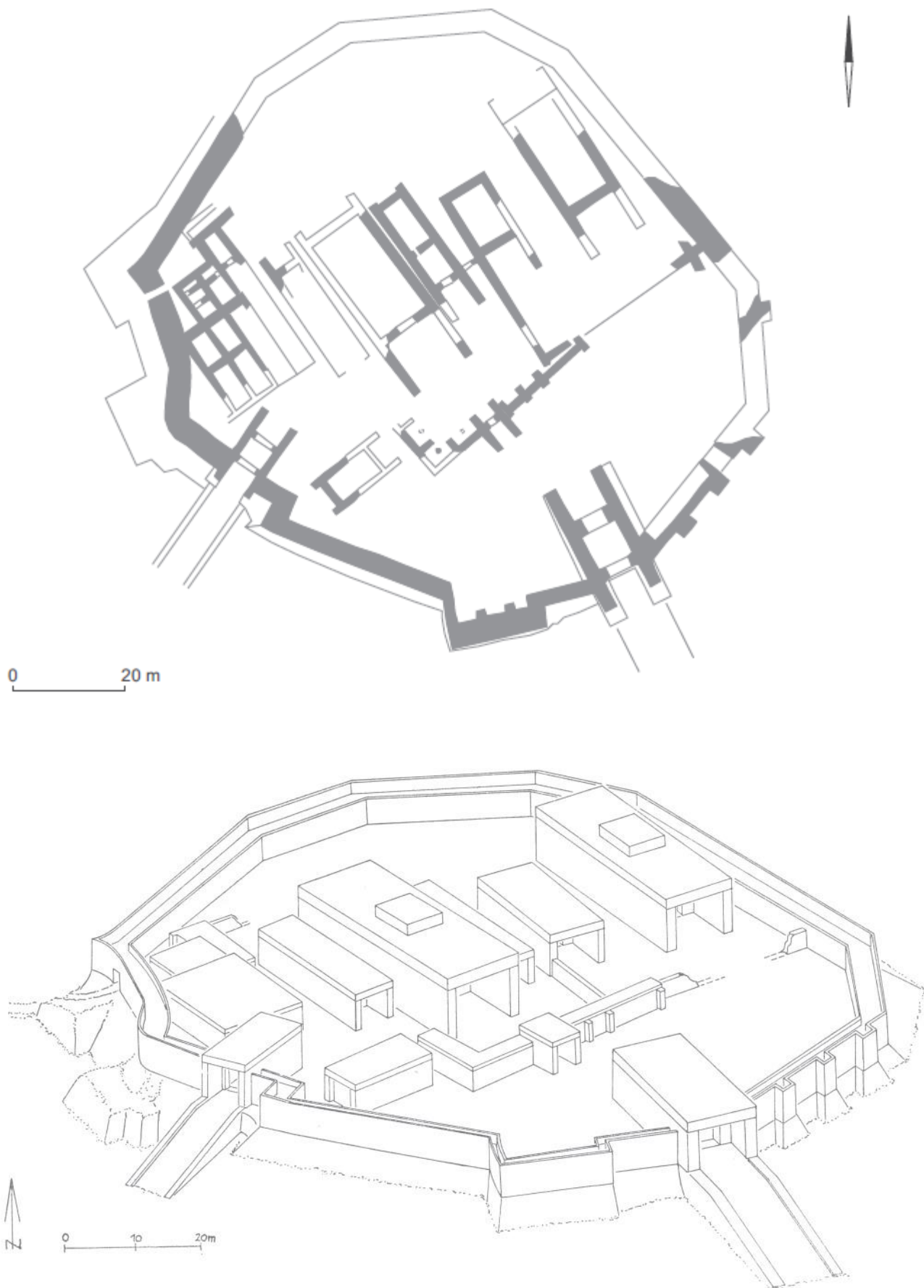
2.9., 2.10. Троя, слой II. План и реконструкция (по Ширмеру)
