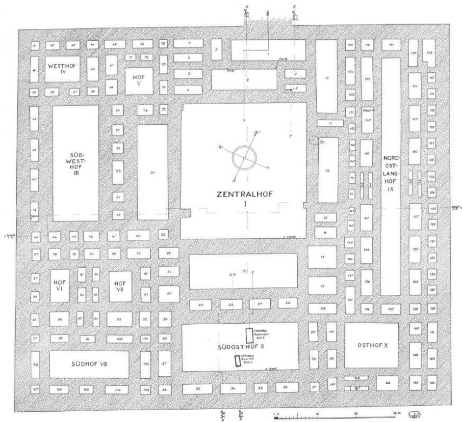
2.17. Ашшур, Старый дворец.
