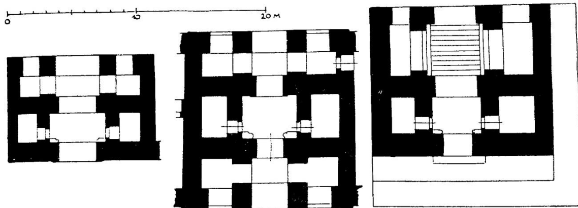
2.21. Структура ворот: склад при Храме 1, Храм 1, Язылыкая
