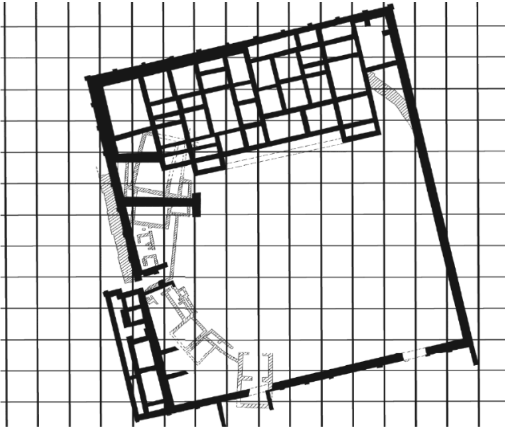
2.15. Кюльтепе, «Дворец Варсамы»
