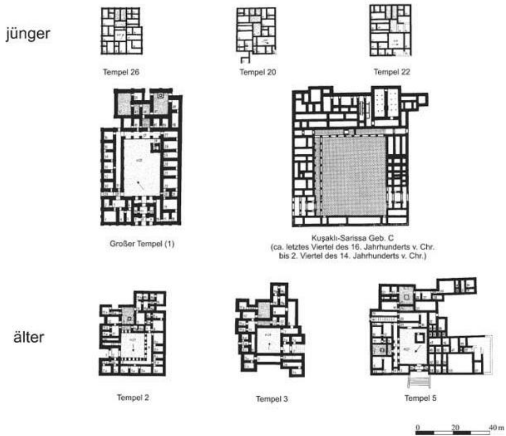
2.19. Планы хеттских храмов – 1, 2, 3, 5, 20, 22, 26 в Богазкее, «Здание С» в Кушаклы
