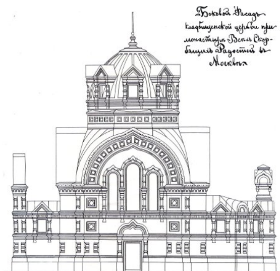
Рис.9. Чертёж храма Трёх Святителей. Боковой фасад
