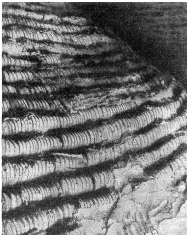
Рис. 12. Сан-Витале в Равенне. Первая половина VI в. Купол из керамических трубок. Вид снаружи (фото Бовини)
