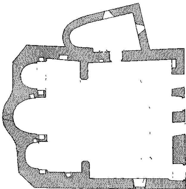
Рис. 12 Церковь Михаила и Гавриила. План и разрез.
